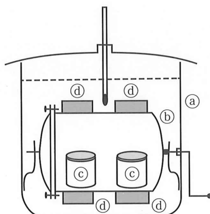
図1 ヘスの熱量計
